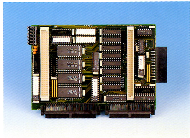
Die VME-Bus Karte mit ROM-Port und Zähler-Logic
